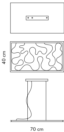
SP S/282 SP S/282 S con specchio/with mirror SP S/282 V con vetro bianco/with white glass STRIP LED 48W CE
