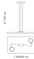
SP 8/280 2 x max 20 W E27 CE
