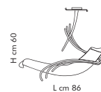
SP 8/230 4 x max 60 W E14
