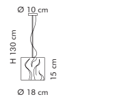
SP 7/238 1 x max 42W ECO E14 CE
