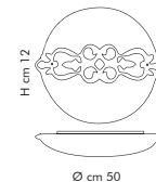
LS 5/258 3 x max 42 W ECO E27
