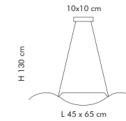
SP 8/244 2 x max 70W ECO E27 or 1 x max 160W ECO R7s 114 mm CE
