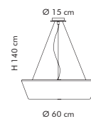
SP 7/241 2 x max 42W ECO E27 CE
