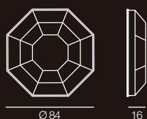
993/8PL-GR-B... Ø 84 x Sp. 16 cm ⦿ E14 8x40W
