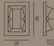
1028/2AP-LN... L 28 x H 38 x Sp. 10,5 cm E14 2x60W
