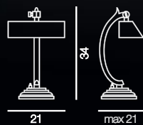
1871/1LU... L 21 x H 34 x Sp. max 21 cm ⊙ E14 1x40W
