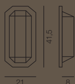
1055/2AP-LN... L 21 x H 41,5 x Sp. 8 cm ● E14 2x40W
