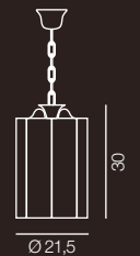
1015/1S-PC... Ø 21,5 x H 30 cm E27 1x60W
