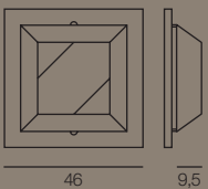
975/4PL-LN... L 46x46 x Sp. 9,5 cm ⦿ E14 4x40W
