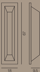
1039/2AP-LN... L 18 x H 67 x Sp. 9,5 cm E14 2x40W
