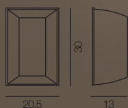
1021/2AP-B... L 20,5 x H 30 x Sp. 13 cm ● E14 2x40W
