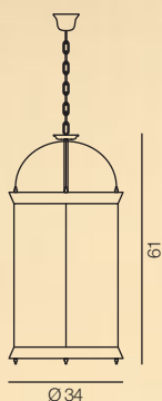
1802/4S-GR-LN... Ø 34 x H 61 cm ○ E14 4x60W
