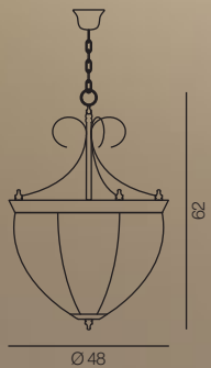
1814/3S-GR-LN... Ø 48 x H 62 cm E14 3x60W
