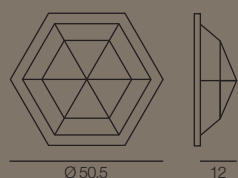
1053/3PL-LN... Ø 50,5 x Sp. 12 cm ⦿ E14 3x40W
