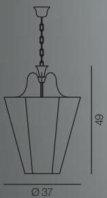
1035/3S-MG... Ø 37 x H 49 cm ⦿ E14 3x60W
