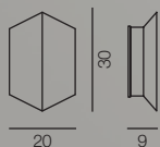
1040/2AP-B... L 20 x H 30 x Sp. 9 cm E14 2x60W
