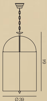
1803/5S-MG... Ø 39 x H 64 cm E14 5x60W
