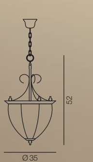
1813/3S-LN... Ø 35 x H 52 cm E14 3x60W
