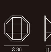
967/2PL-LN... Ø 36 x Sp. 11,5 cm ⦿ E14 2x40W
