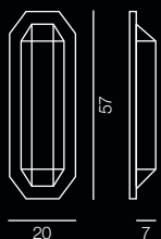
1037/2AP-LN... L 20 x H 57 x Sp. 7 cm E14 2x40W
