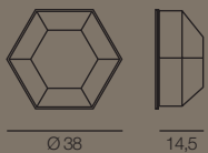
966/3PL-B... Ø 38 x Sp. 14,5 cm E27 3x40W ES
