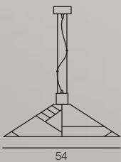
3055/1S... L 54x54 x H max 106 cm E27 1x75W ES
