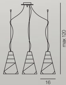
3052/3S... L 16x16 x H max 120 cm E14 3x60W ES
