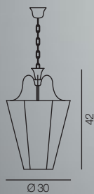
1035/1S-GR... Ø 30 x H 42 cm ⦿ E27 1x60W
