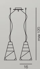
3051/2S... L 16x16 x H max 120 cm E14 2x60W ES
