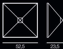
1113/4PL-MD... L 52,5 x Sp. 23,5 cm E27 4x40W ES
