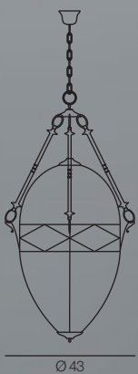
2077/5S... Ø 43 x H 84 cm ○ E14 5x60W
