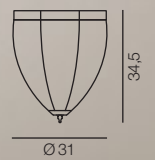
1816/3PL-B... Ø 31 x H 34,5 cm E14 3x40W
