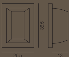
1021/2AP-LN... L 26,5 x H 36,5 x Sp. 13 cm ● E14 2x40W
