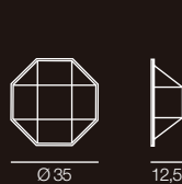
968/2PL-B... Ø 35 x Sp. 12,5 cm ⦿ E14 2x40W
