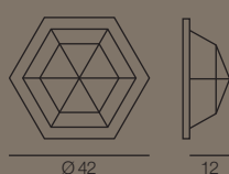
1054/3PL-LN... Ø 42 x Sp. 12 cm ⦿ E14 3x40W
