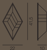
950/2AP-B... L 22 x H 41,5 x Sp. 10 cm ● E14 2x40W
