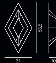
2016/2AP-LN... L 31 x H 56,5 x Sp. 10 cm E14 2x40W
