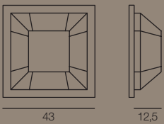
2009/4PL-LN L 43x43 x Sp. 12,5 cm E14 4x40W
