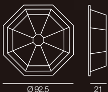
1025/8PL-GR-LN... Ø 92,5 x Sp. 21 cm ⦿ E14 8x40W
