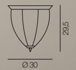
1815/1PL-LN... Ø 30 x H 29,5 cm E27 1x75W
