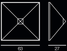
1114/5PL-GR... L 63 x Sp. 27 cm E27 5x40W ES
