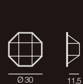
967/2PL-B... Ø 30 x Sp. 11,5 cm ⦿ E14 2x40W
