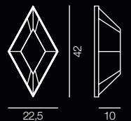
2016/2AP-B... L 22,5 x H 42 x Sp. 10 cm E14 2x40W
