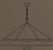
1005/1S-MG... Ø 70 x H 23,5 cm E27 1x60W ES
