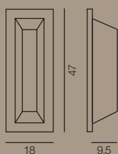
1038/2AP-LN... L 18 x H 47 x Sp. 9,5 cm E14 2x40W
