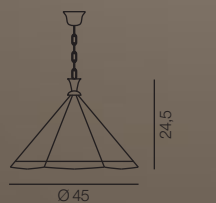
1005/1S-MD... Ø 45 x H 24,5 cm E27 1x60W ES
