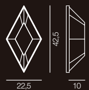
2010/2AP-B... L 22,5 x H 42,5 x Sp. 10 cm E14 2x40W
