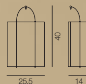
1805/2AP-B... L 25,5 x H 40 x Sp. 14 cm E14 2x60W
