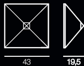
1112/4PL-PC... L 43 x Sp. 19,5 cm E27 4x40W ES
