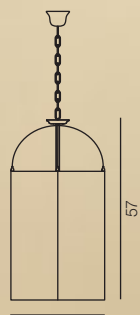
1802/4S-GR... Ø 31 x H 57 cm E14 4x60W
