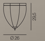
1815/1PL-B... Ø 26 x H 29,5 cm E27 1x75W
