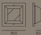
974/2PL-LN... L 36,5x36,5 x Sp. 9,5 cm ⦿ E14 2x40W
