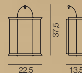
1804/1AP-LN... L 22,5 x H 37,5 x Sp. 13,5 cm ○ E14 1x60W
