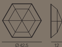
1053/3PL-B... Ø 42,5 x Sp. 12 cm ⦿ E14 3x40W
