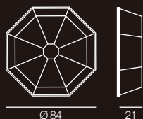
1025/8PL-GR-B... Ø 84 x Sp. 21 cm ⦿ E14 8x40W
