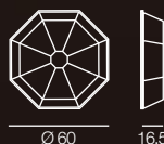
1025/4PL-GR-B... Ø 60 x Sp. 16,5 cm ⦿ E14 4x40W
