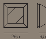
974/2PL-B... L 29,5x29,5 x Sp. 9,5 cm ⦿ E14 2x40W
