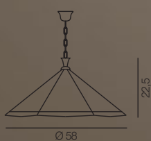
1005/1S-GR... Ø 58 x H 22,5 cm E27 1x60W ES
