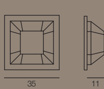
2008/2PL-LN L 35x35 x Sp. 11 cm E14 2x40W
