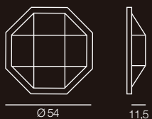
969/4PL-LN... Ø 54 x Sp. 11,5 cm ⦿ E14 4x40W
