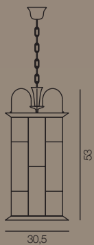
1030/4S-GR-LN... L 30,5x30,5 x H 53 cm E14 4x60W
