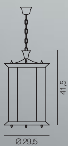
1070/1S-LN... Ø 29,5 x H 41,5 cm E27 1x60W
