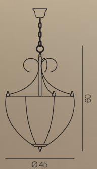
1814/3S-GR... Ø 45 x H 60 cm E14 3x60W
